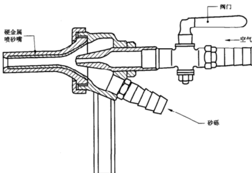
图2 典型的喷射系统
